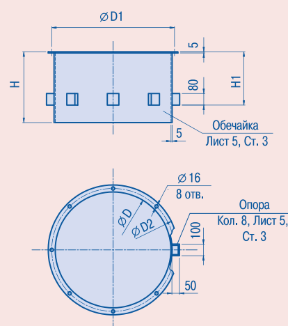
Рис. 2 Эскиз стакана
